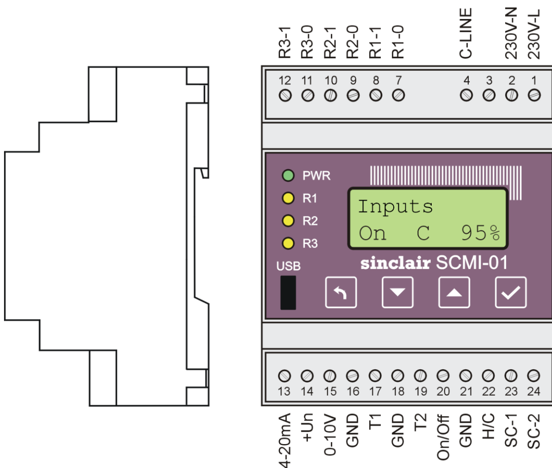
Fig. 1. SCMI-01.5 control module
