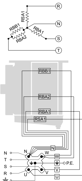
Connexion 400V/3/50-60Hz PRÉDISPOSÉE
