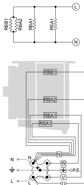
Connexion 230V/1/50-60Hz à prédisposer
