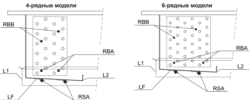
Расположением электрических ТЭНов оттайки
