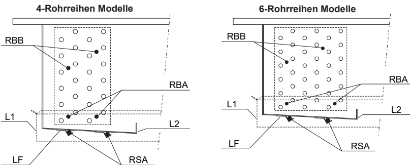
Einzelheit der Heizstäbebefestigung
