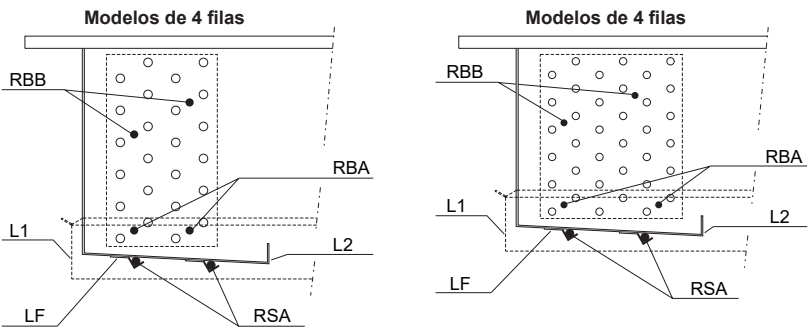
Detalle de la posición de las resistencias
