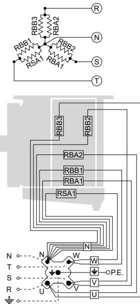
Connexion 400V/3/50-60Hz PRÉDISPOSÉE
