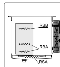
Détail de pos. résistances
