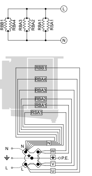
Подключение 230V/1/50-60Hz для подготовки
